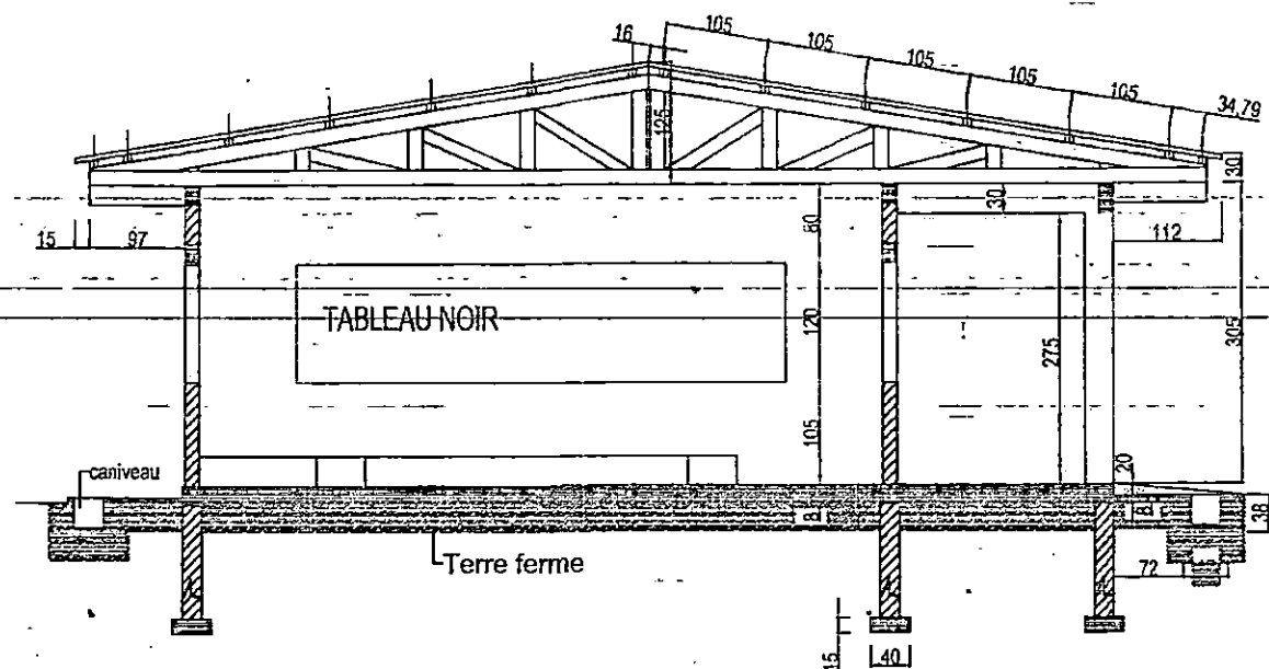
COUPE A-A
