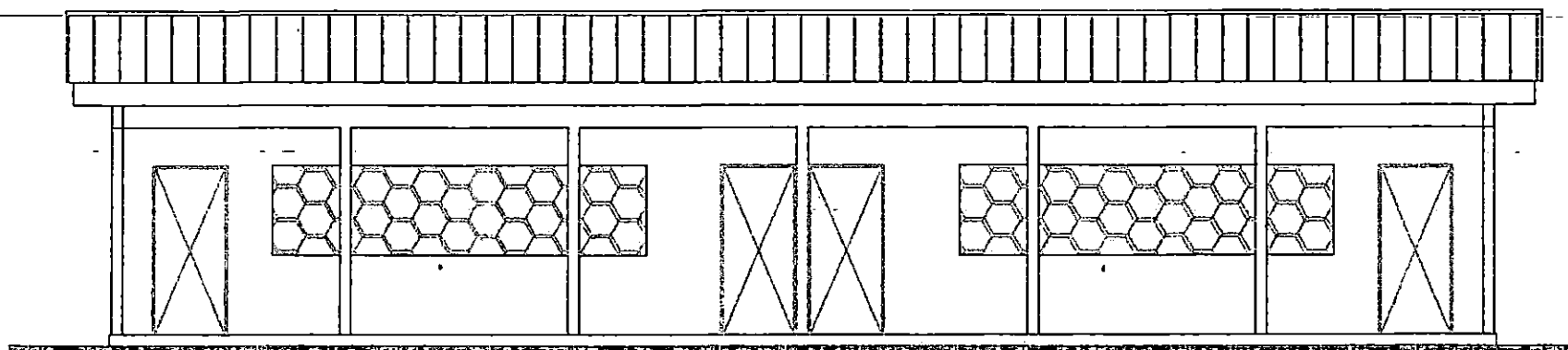
FACADE PRINCIPALE
